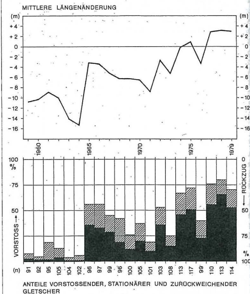
LÄNGENÄNDERUNG DER ÖSTERR. GLETSCHER 1959 - 1979
