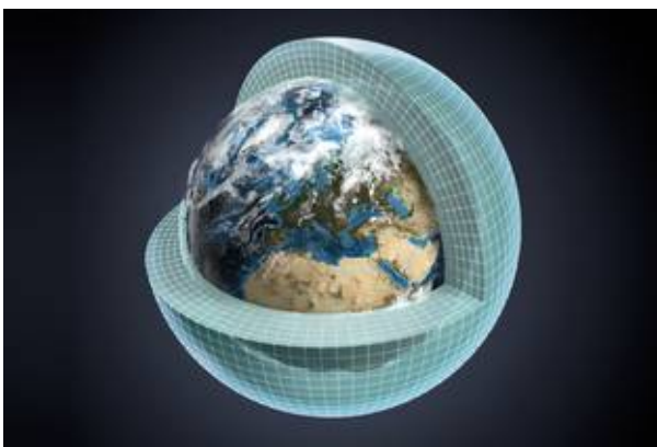
Symbolbild Klimamodellierung (Grafik: Martin Künsting)
