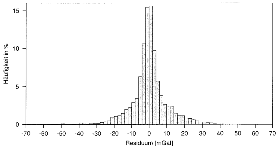
Abbildung 4.7: Häufigkeitsverteilung der Residuenwerte im gesamten Modell.
