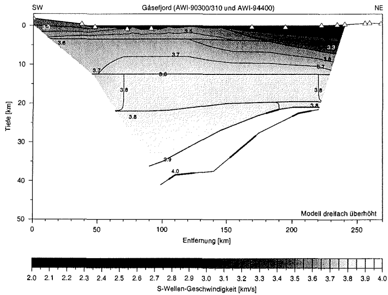
Abbildung 3.10: Geschwindigkeitsmodell der S-Wellen für das Profil Gåsefjord. Weitere Erläuterungen siehe Abb. 3.7.
