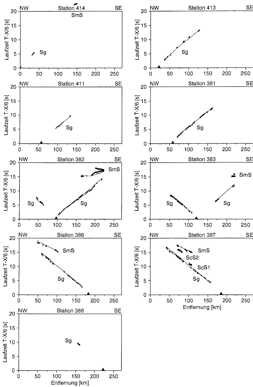
Abbildung 3.24: Laufzeiten der S-Wellen für das Profil Nordvestfjord. Weitere Erläuterungen siehe Abb. 3.5.
