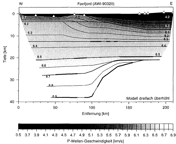
Abbildung 3.14: Geschwindigkeitsmodell der P-Wellen für das Profil Føn fjord. Weitere Erläuterungen siehe Abb. 3.7.
