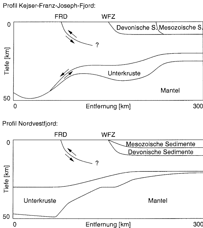
Abbildung 5.2: Schematische Darstellung der paläozoisch-mesozoischen Extensionsstrukturen in Anlehnung an das Modell von Schlindwein (1998). FRD: Fjord Region Detachment . WFZ: Western Fault Zone . S.: Sedimente. Die Pfeile geben die Bewegungsrichtungen der einzelnen Krustenblöcke während des devonischen Extensionskollapses an. Längen sind nicht maßstabsgetreu.
