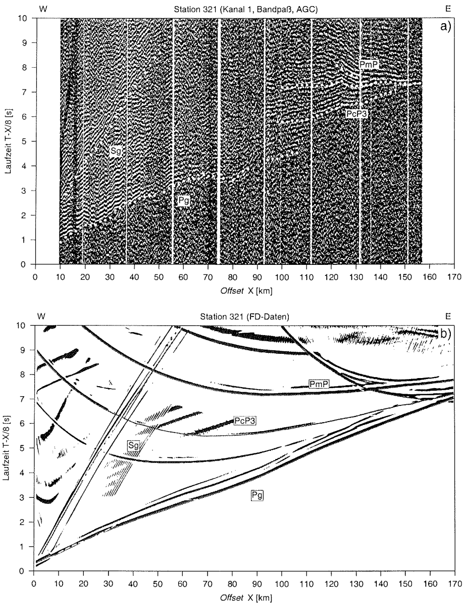
Abbildung B.2: Seismogrammausschnitt der Station 321 des Profils Føn fjord. a) Reale Daten. Abgelesene Einsätze sind markiert und beschriftet. b) Mit FD modellierte Daten. Wichtige Phasen sind markiert und beschriftet. Die unterbrochenen Linien stellen die mit Raytracing berechneten Laufzeitkurven dar.
