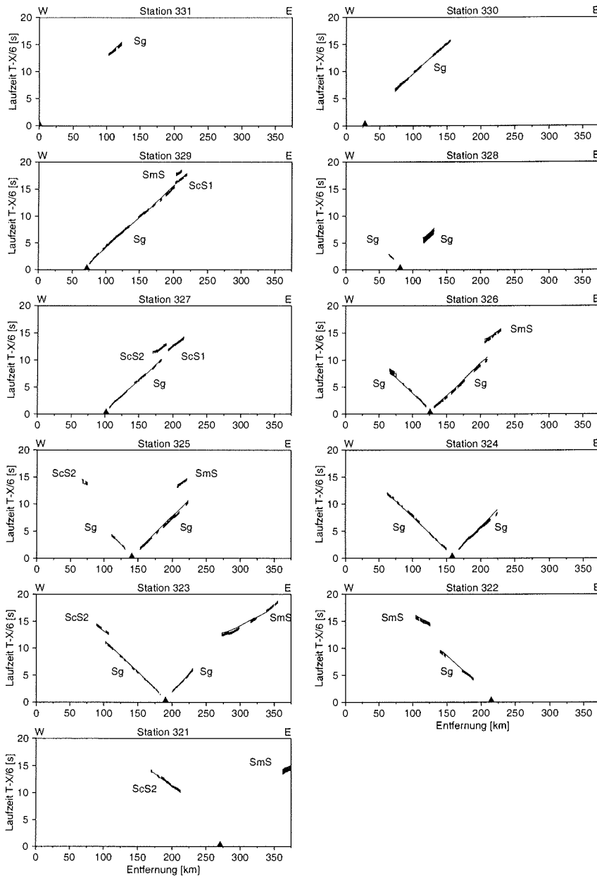
Abbildung 3.37: Laufzeiten der S-Wellen für das Profil Keiser-Franz-Joseph-Fjord. Weitere Erläuterungen siehe Abb. 3.5.
