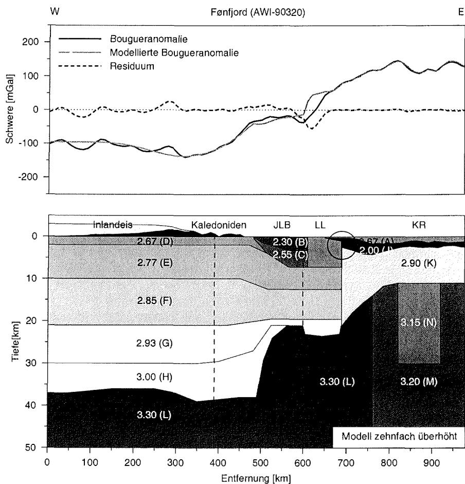
Abbildung 4.2: Dichtemodell für das Profil Føn fjord. JLB: Jameson-Land-Becken. LL: Liverpool-Land. KR: Kolbeinsey-Rücken. Die Bouguerschwere, die modellierte Bouguerschwere und das Residuum sind als Kurven dargestellt. Die Dichtewerte und Abkürzungen der modellierten Schichten sind angegeben. Unterbrochene Linien umrahmen das tiefenseismische Profil. Der Kreis markiert den Bereich der fehlerhaften Sedimentmächtigkeiten. Die nicht im Modell enthaltene Oberflächentopographie ist schematisch dargestellt. Das Profil ist zehnfach überhöht.
