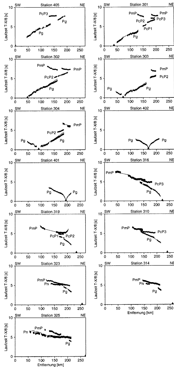
Abbildung 3.5: Laufzeiten der P-Wellen für das Profil Gåsefjord. Abgelesene Laufzeiten sind mit ihren Fehlerbalken dargestellt. Durchgezogene Linien zeigen die modellierten Laufzeitkurven. Schwarze Dreiecke markieren die Lage der Stationen.
