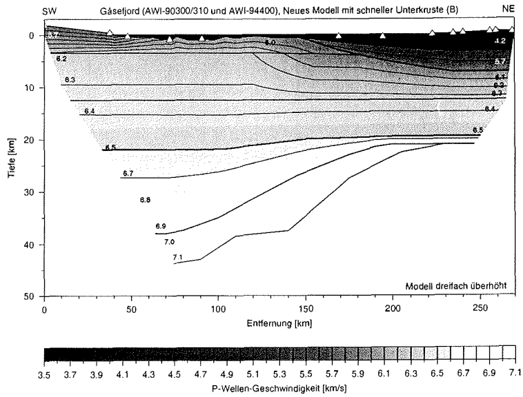
Abbildung 3.63: Geschwindigkeitsmodell der P-Wellen für das Profil Gåsefjord mit schneller Unterkruste (B). Weitere Erläuterungen siehe Abb. 3.7.
