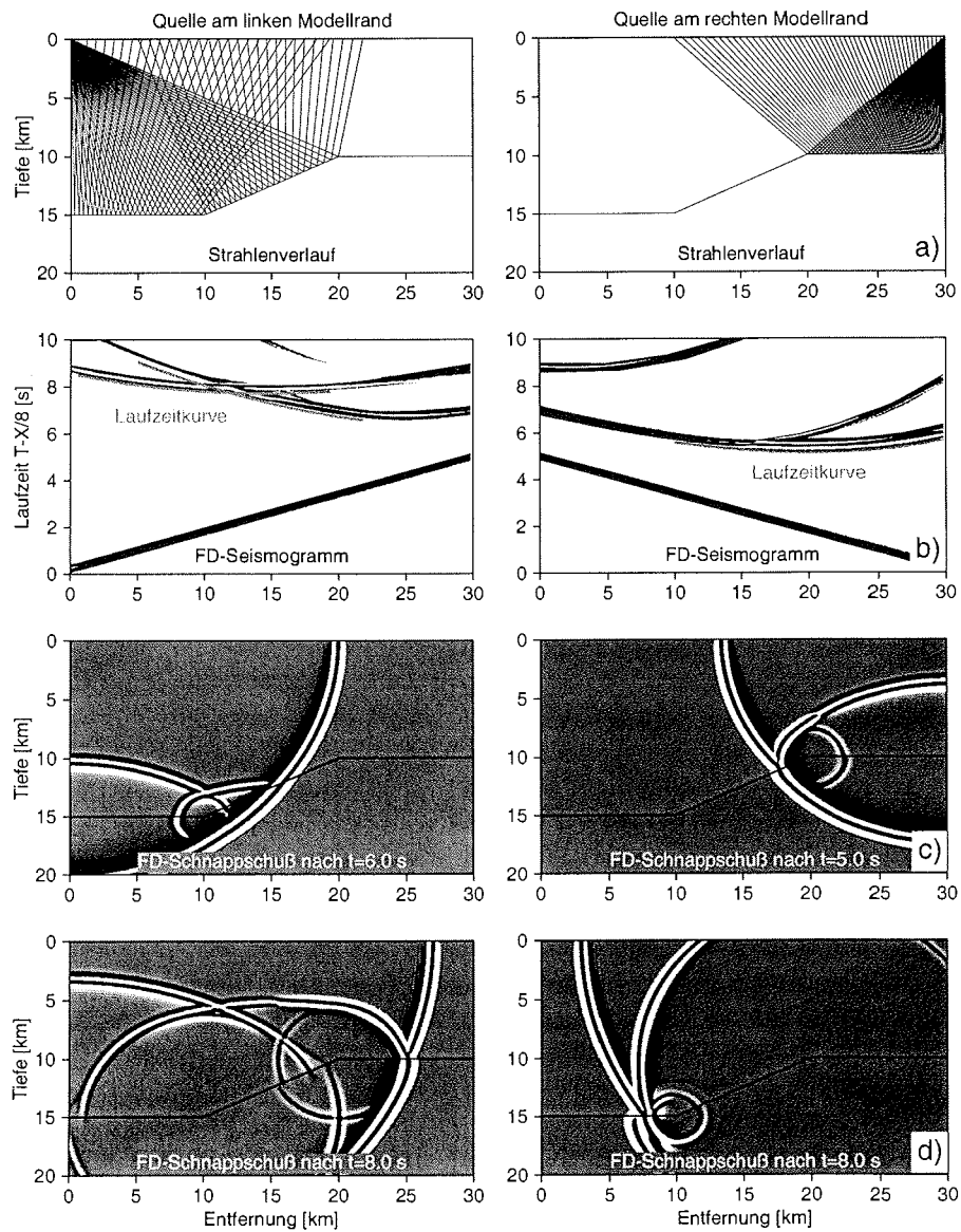
Abbildung 3.57: Diffraktion an einer Kante. a) Mit Raytracing berechnete Strahlen. b) Mit FD modelliertes Seismogramm. Die durchgezogenen Linien stellen die mit Raytracing berechneten Laufzeitkurven für die Reflexionen dar. c) und d) FD-Schnappschüsse mit Diffraktionen zu unterschiedlichen Zeitpunkten.
