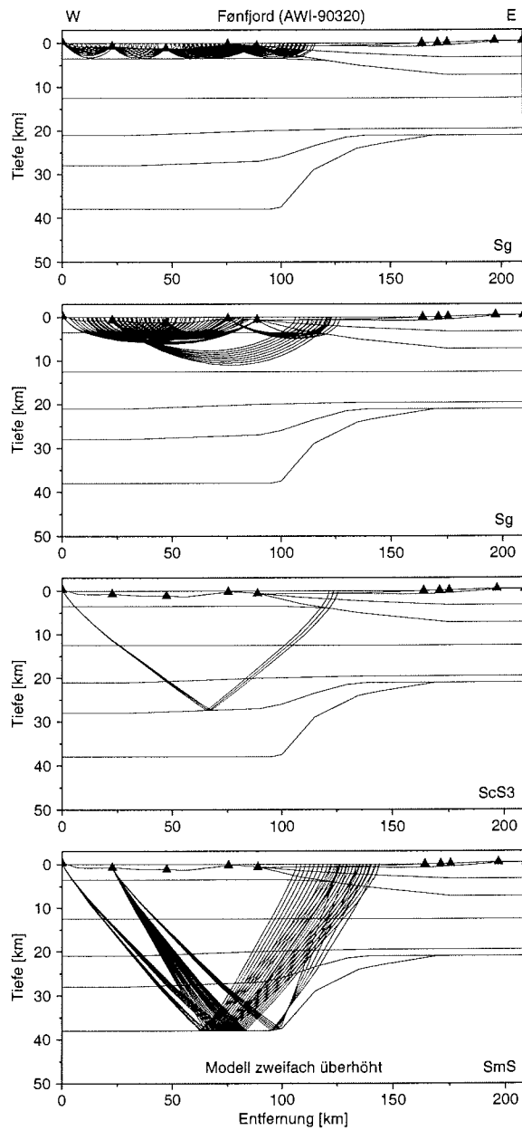
Abbildung 3.16: Strahlenverlauf der S-Wellen für das Profil Fønford. Weitere Erläuterungen siehe Abb. 3.6.
