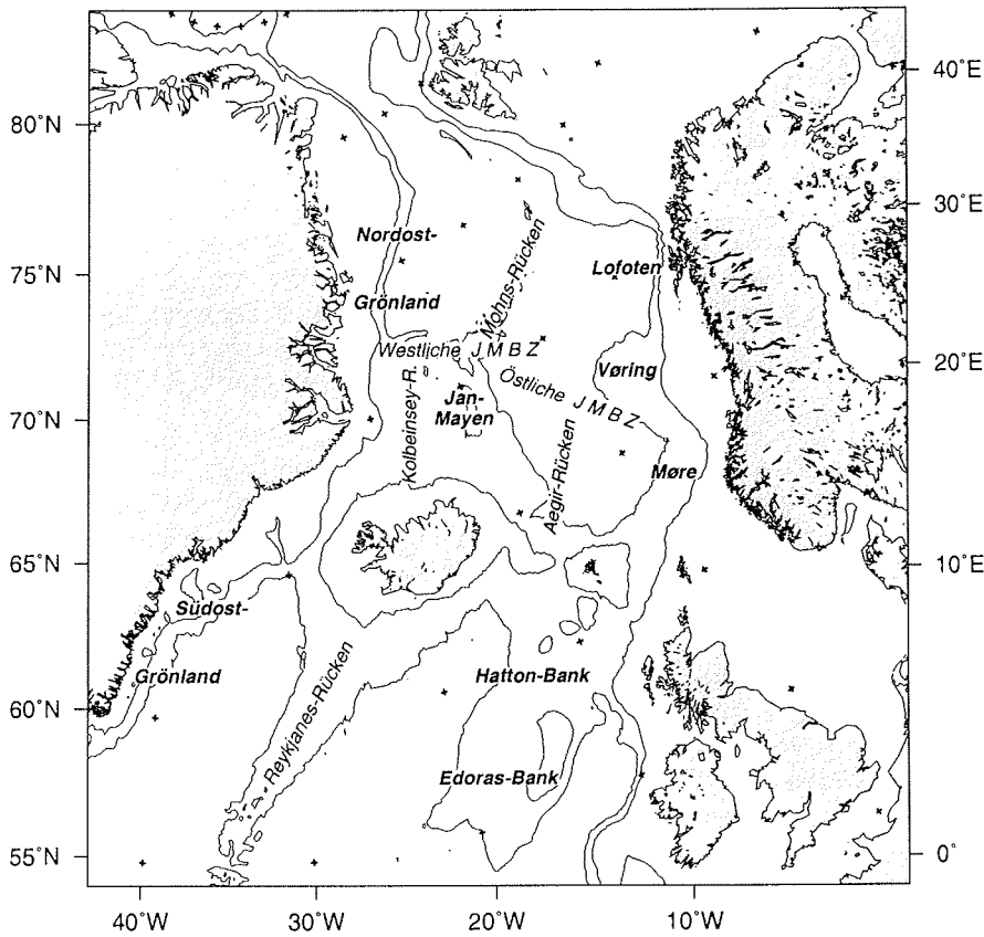
Abbildung 5.3: Kontinentalränder des nördlichen Atlantiks. JMBZ: Jan-Mayen-Bruchzone. R.: Rücken. Die 0.5km und 2.0km Isolinien stellen die vereinfachte Bathymetrie dar. Wichtige Rücken und Bruchzonen sind beschriftet.
