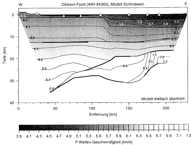
Abbildung 3.46: Geschwindigkeitsmodell der P-Wellen für das Profil Dickson-Fjord nach Schindwein (1998). Weitere Erläuterungen siehe Abb. 3.7.
