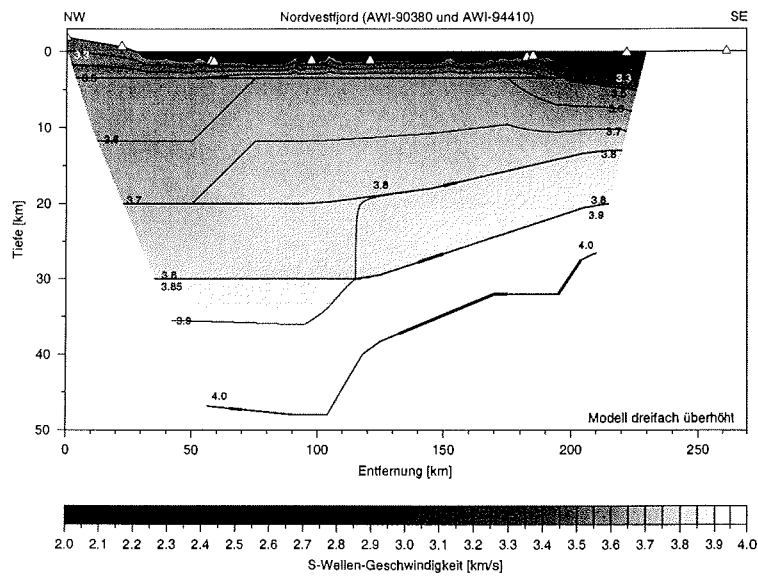
Abbildung 3.26: Geschwindigkeitsmodell der S-Wellen für das Profil Nordvestfjord. Weitere Erläuterungen siehe Abb. 3.7.
