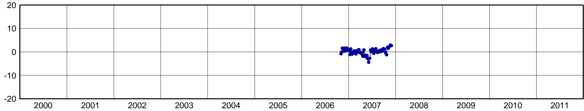
TUMA-North Component [mm]
