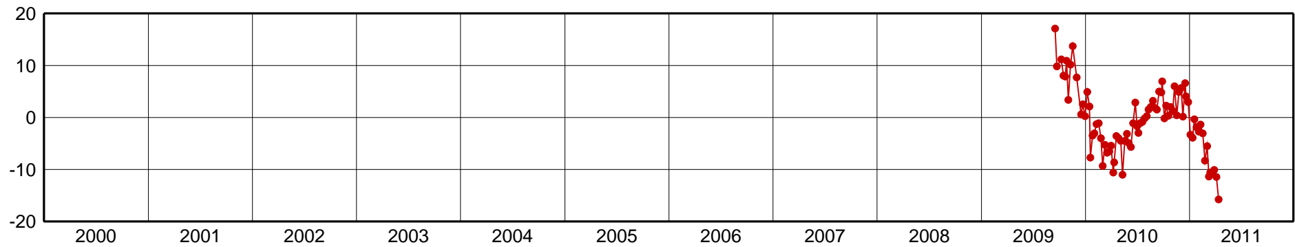
SJRP-Up Component [mm]
