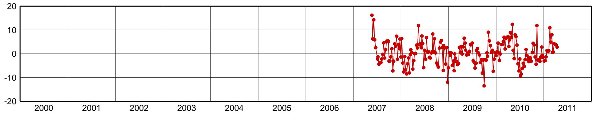
SMRT-Up Component [mm]
