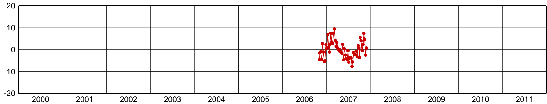
TUMA-Up Component [mm]
